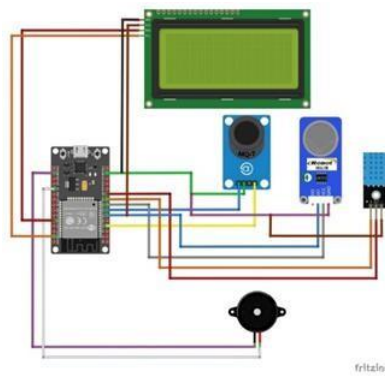
Gambar 3. Rangkaian Komponen
