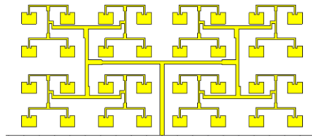
d. Array 8 x 4
