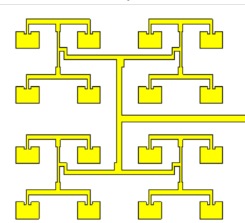
c. Array 4 x 4
