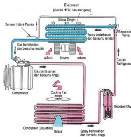
Gambar 3 Cara Kerja AC
