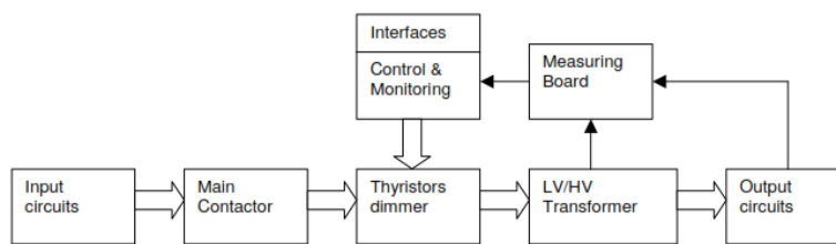
Gbr. 2. Blok Diagram CCR AUGIER DIAM 4000
