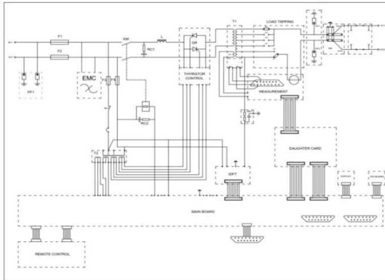
Gbr. 1 Rangkaian sistem secara keseluruhan CCR AUGIER DIAM 4000
