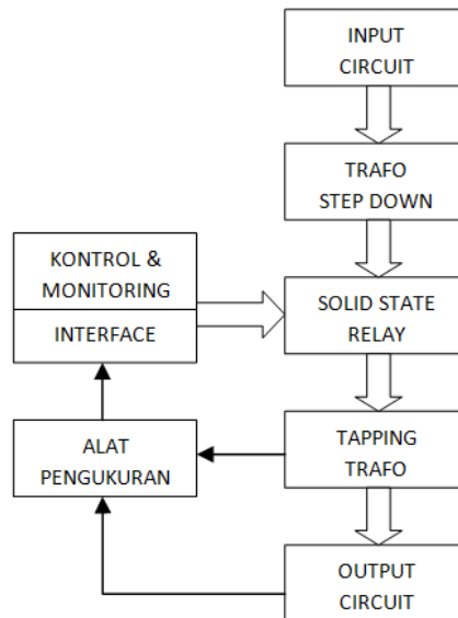
Gbr.5. Blok Diagram Rancangan
